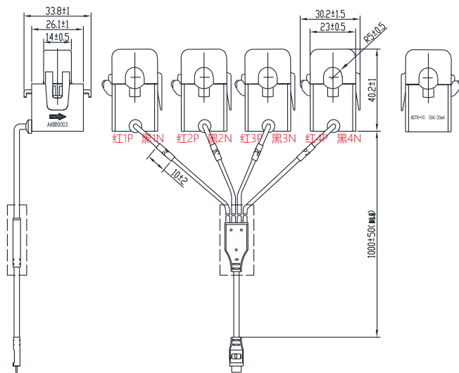
NTCK-10(50A*4) (一拖四)
