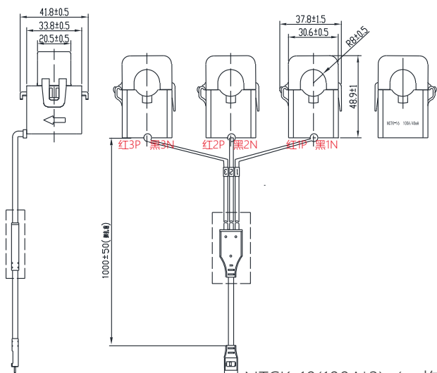
NTCK-10(100A*3) (一拖三)
