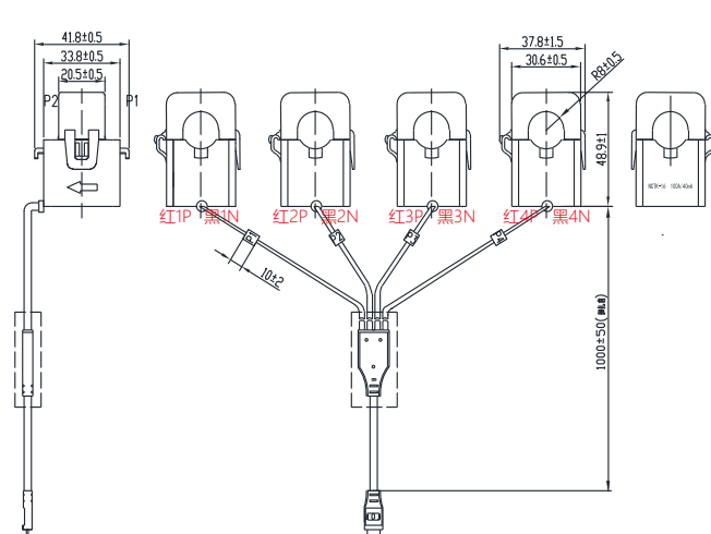
NTCK-10(100A*4) (一拖四)
