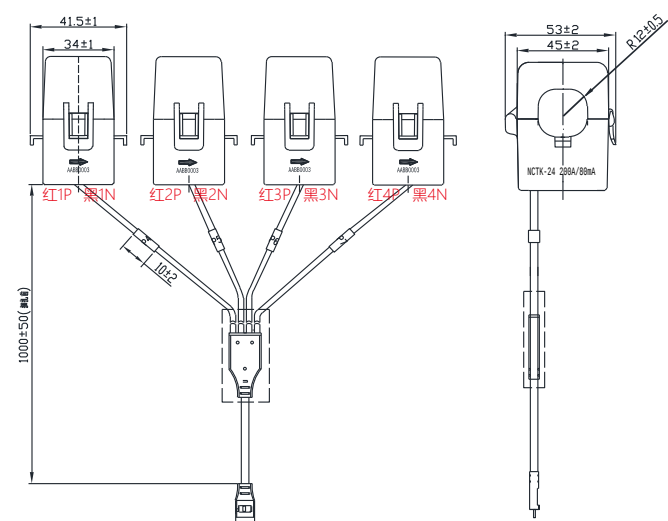
NTCK-10(200A*4) (一拖四)
